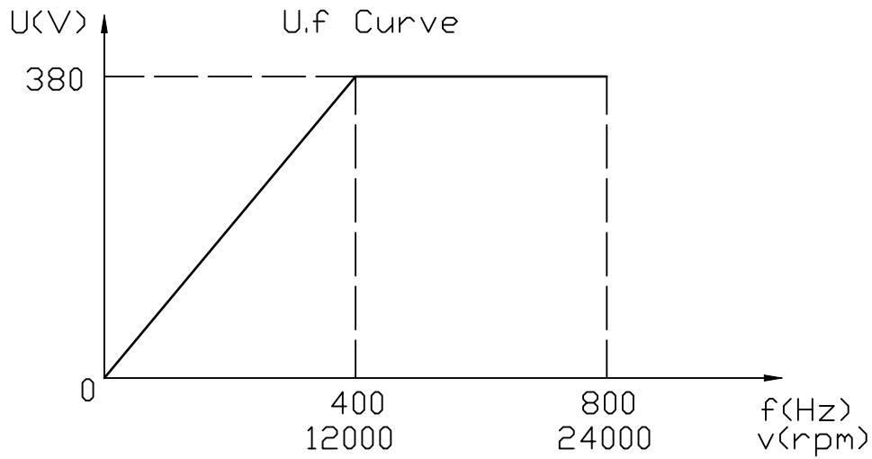
频压曲线
